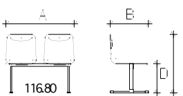
Várótermi pad / Gestühl für den Wartesaal / Waiting room seating
